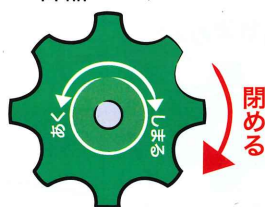
容器バルブ
